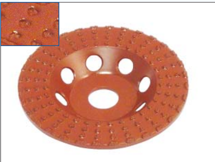
DIAMANT-Raspeltopf DRT-125, BRAUN, Art.-Nr. 223.253 zum Anschleifen von glatten PU-/Acrylbelägen, Abschleifen von Kleberschichten auf Holz- oder harten Untergründen, aufgespritzter Fahrbahnmarkierungen
